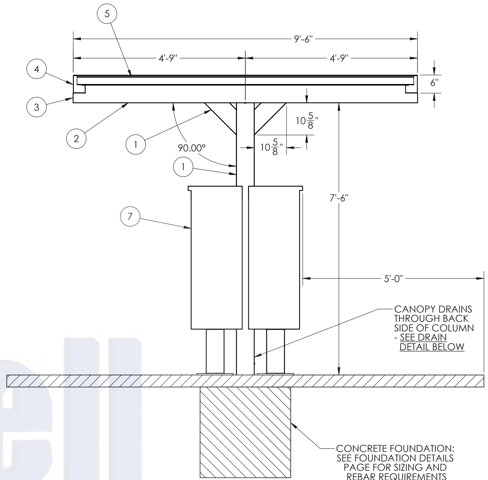
SECTION A-A SCALE 1 : 19
